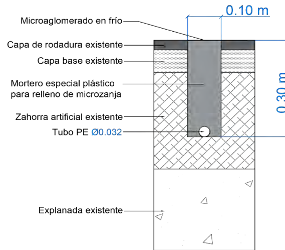
Figura 5. Esquema de microzanja en pavimento.
