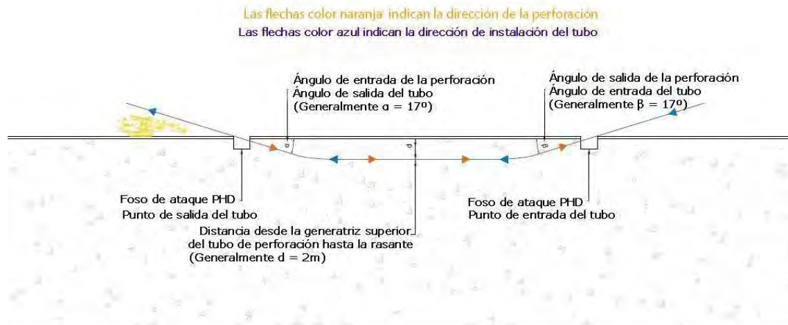
Figura 6. Esquema de perforación e instalación del tubo cruzamiento en la carretera N-623.
