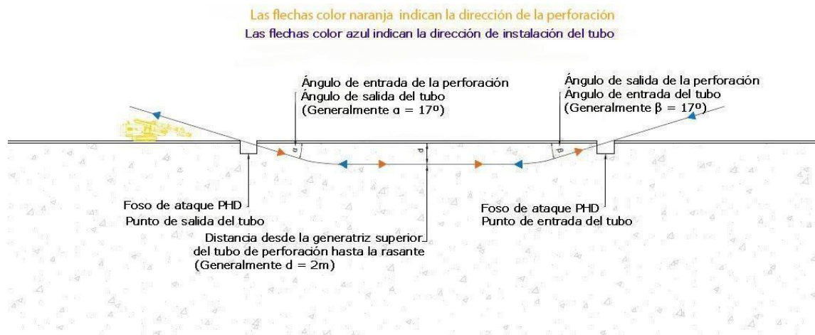
Figura 6. Esquema de perforación e instalación del tubo cruzamiento en las carreteras SC-BU-24 y CL-269
