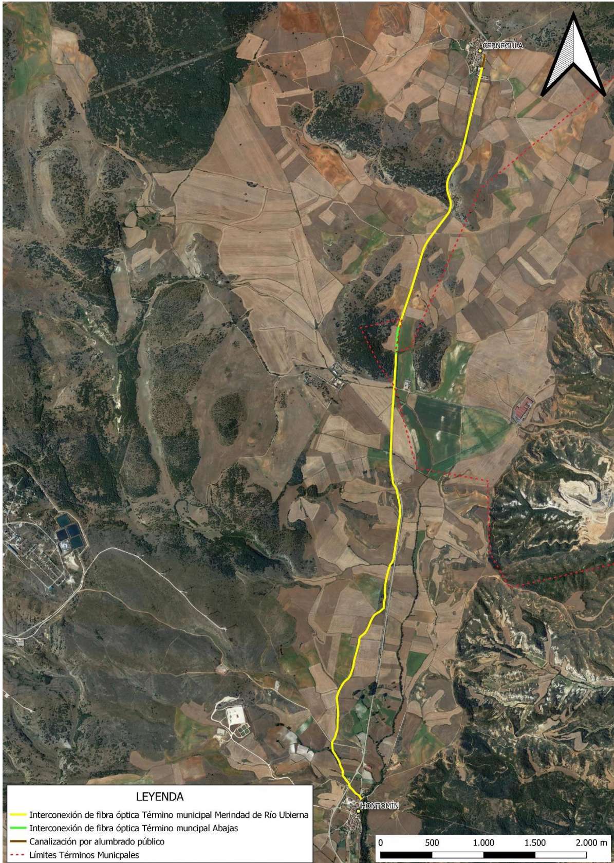
Figura 1. Trazado de la instalación.
